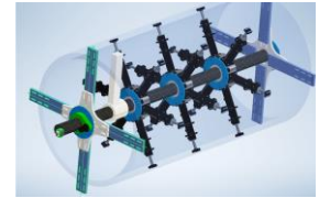
Máy doa lỗ di động
